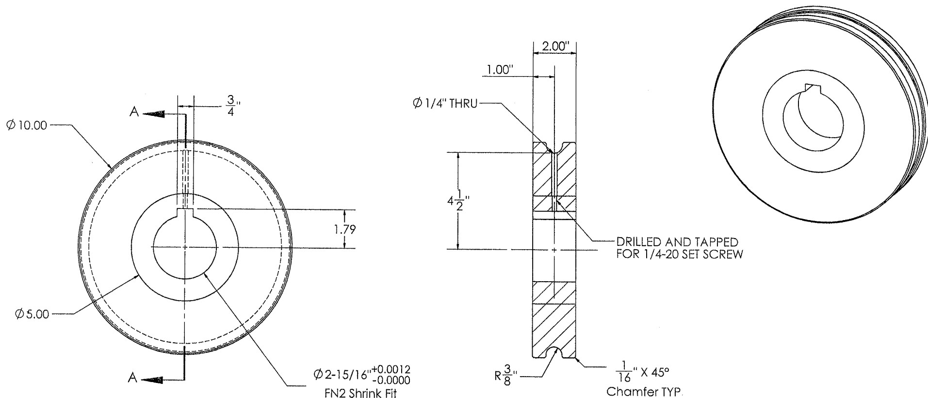
SECTION A-A
